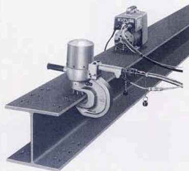
油圧パンチャー A07-1624B
