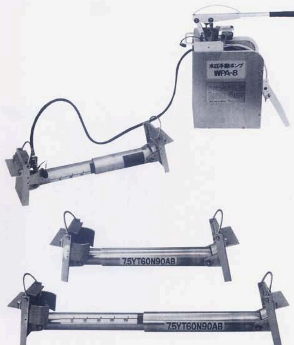
●腹起し・水圧ジャッキ
