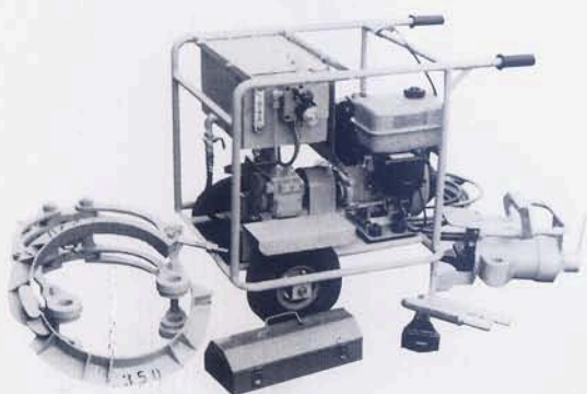
●パイルカッター
