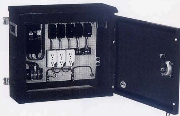
●配電盤
