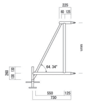
SR750 アウトリガー
