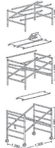
VXW (板ダブル) 2段例
