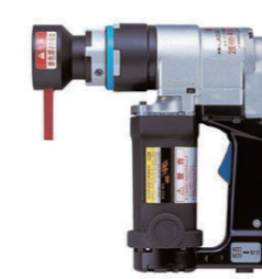
ナット回転角法用1次締レンチ TONE KR-221A
