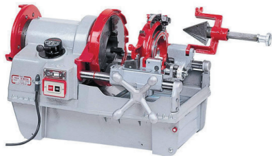
パイプねじ切旋盤 N100A (4インチ) 他
