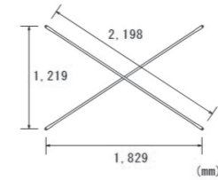
A14 筋交 他各種
