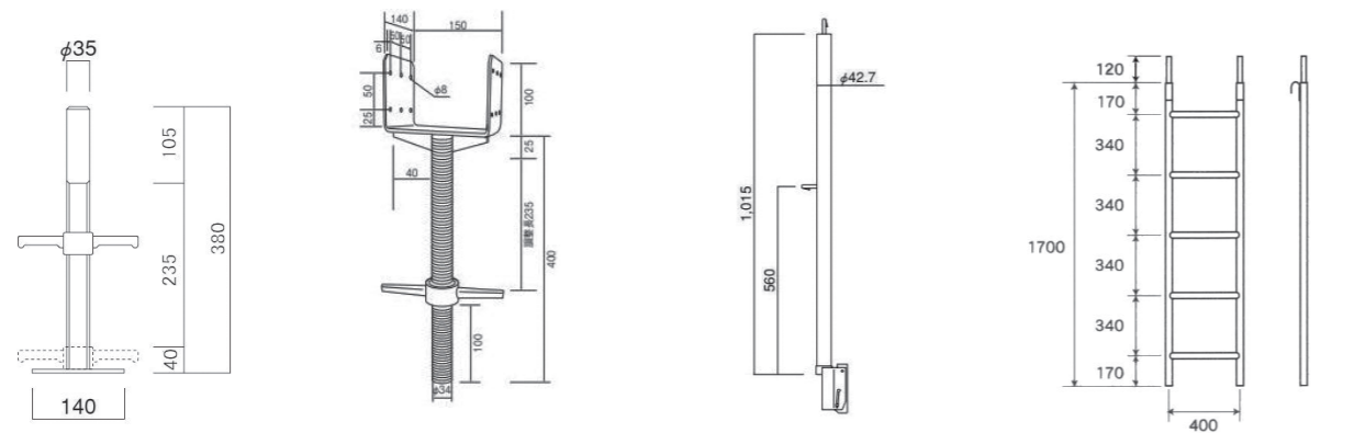
ジャッキベース 各種 大引受ジャッキ LP1000 ビティール用支柱 ビティール用モンキータラップ 各種
