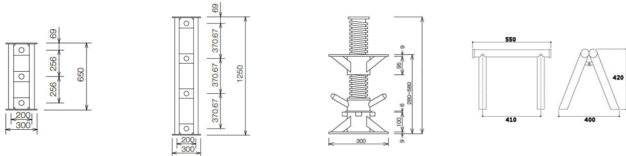
四角支柱 SSH-65 四角支柱 SSH-125 四角支柱 SSJ-58 パイプ馬
