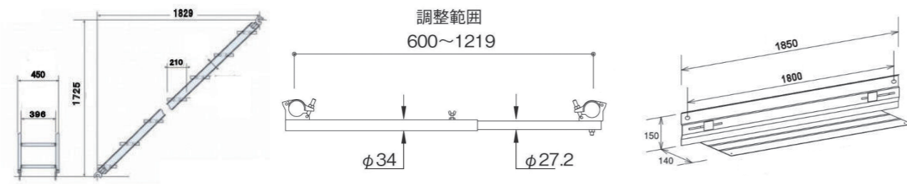
アルミ階段 450 幅 ビティール用 エンドストッパー FN-18 巾木 1800 ビティール用
